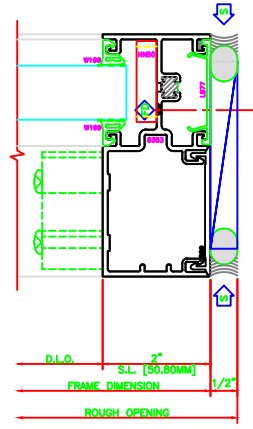
405 LEFT JAMB S433
