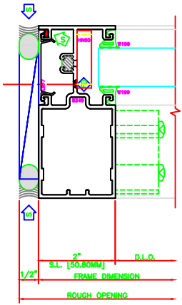
402 LEFT JAMB S433
