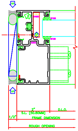
404 LEFT JAMB S433
